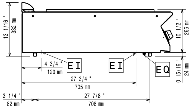
Zij aanzicht
