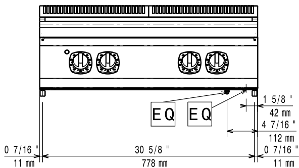
Front aanzicht
